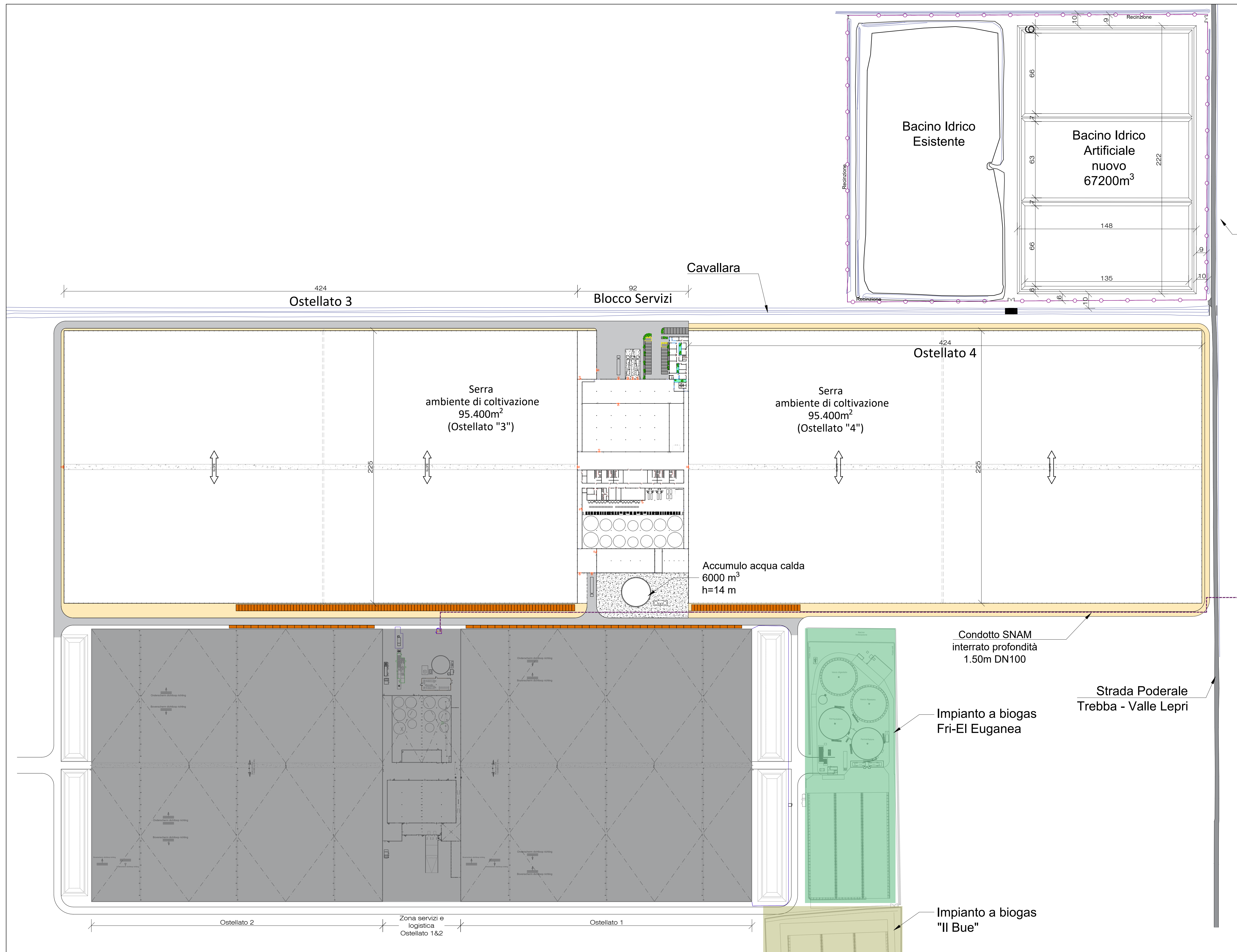
PLANIMETRIA GENERALE STATO DI PROGETTO Scala 1:1500
