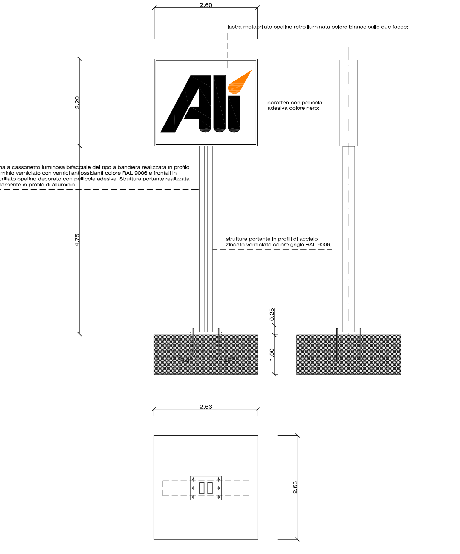
PARTICOLARI INSEGNA PUBBLICITARIA scala 1:50
