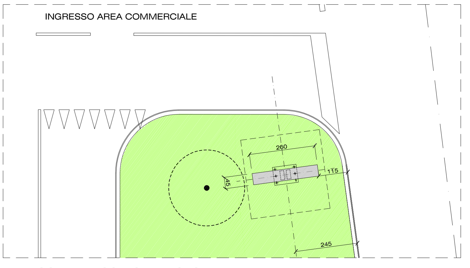
PARTICOLARE POSIZIONE INSEGNA scala 1:50
