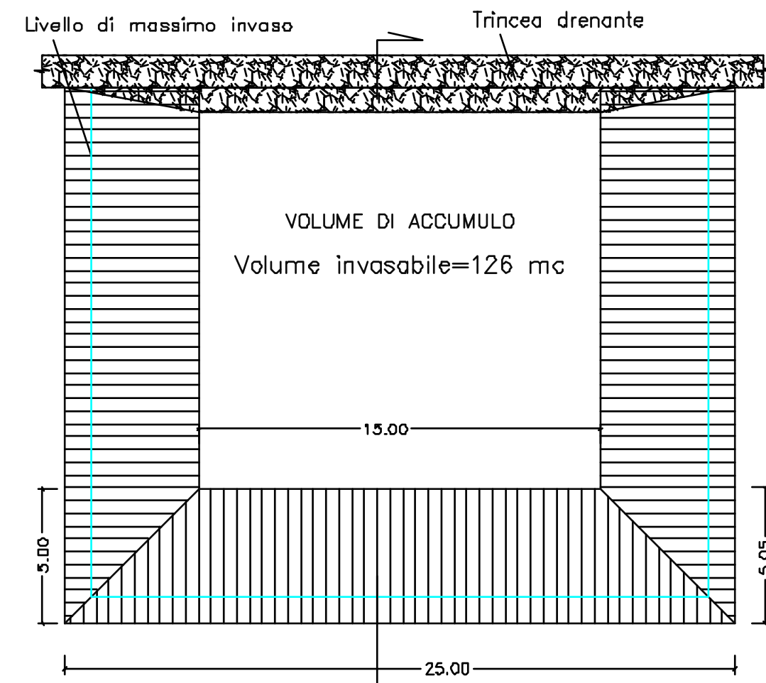
Pianta vasca di accumulo Scala 1:200
