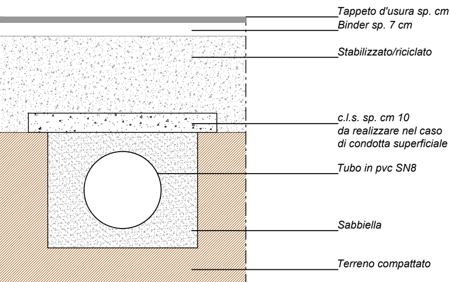
PARTICOLARE ACQUE NERE/BIANCHE scala 1:20
