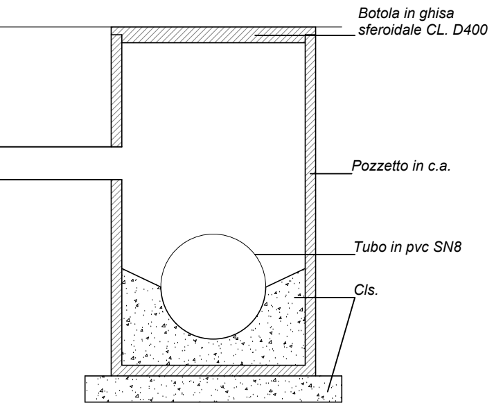
PARTICOLARE POZZETTO ACQUE NERE/BIANCHE scala 1:20
