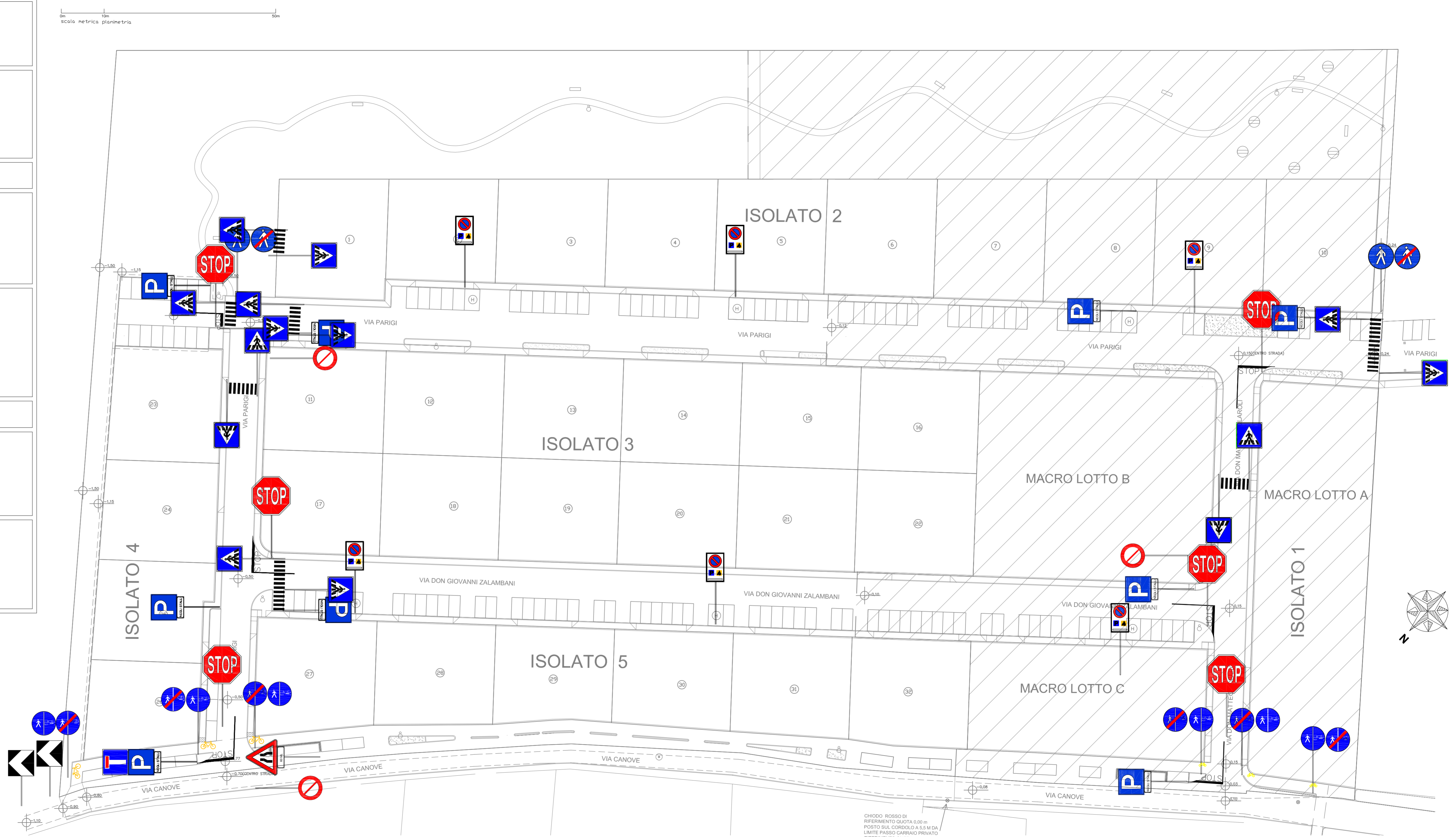
planimetria segnaletica stradale scala 1:500
