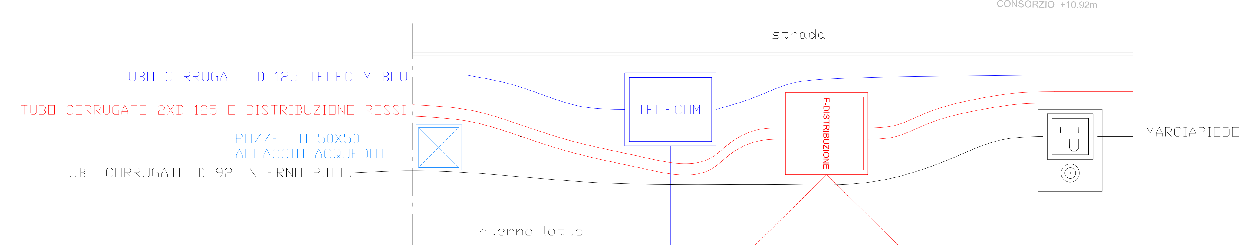
PLANIMETRIA RETE E-DISTRIBUZIONE E TELECOM SC 1:250
