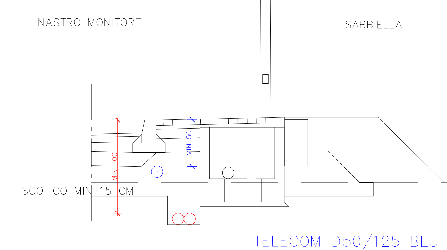
N. 2 CORRUGATI DOPPIA CAM. D 125 ROSSI
