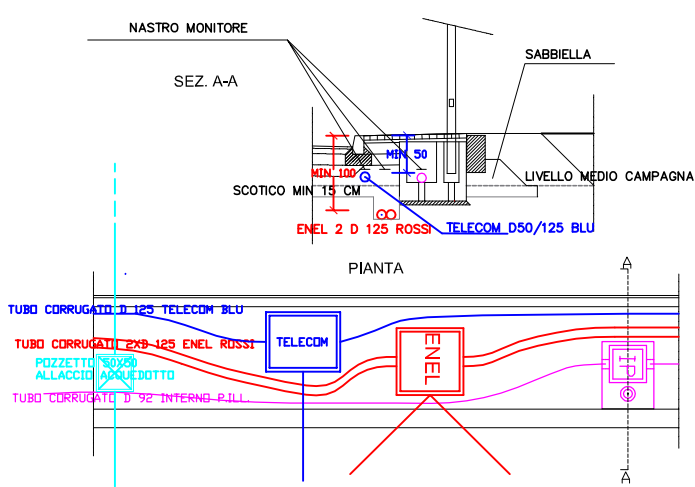
PARTICOLARE TIPO RETE ENEL E TELECOM SC 1:25
