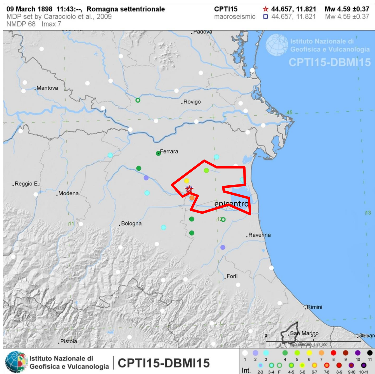
Fig. 5/13: evento del 1898: Romagna Settentrionale. Scala Libera, epicentro ed area in esame.
