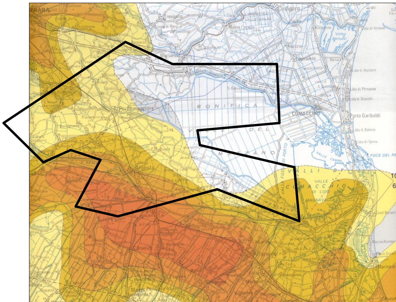
Fig. 6/21: Spessore cumulativo dell'acquifero B. Scala Libera.
