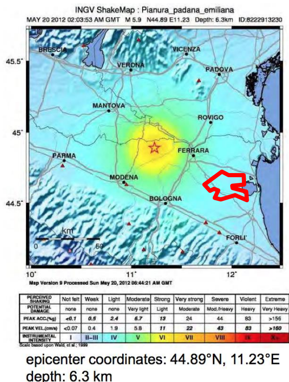
Fig. 5/18: Ubicazione degli epicentri degli eventi del 20 maggio 2012 e sviluppo areale delle relative intensità; il quadratino riporta l'area in esame, Scala libera (immagini tratte da L. Martelli- SGS Regione Emilia- Romagna; 7th Euregeo, Bologna 12- 15 Giugno 2012). Scala Libera.
