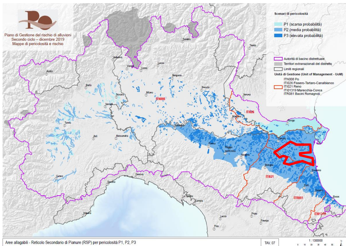
Tav. 6/14: Carta delle Aree Allagabili del Reticolo Secondario di Pianura del Piano di Gestione del Rischio Alluvioni, Secondo Ciclo, Dicembre 2019. Scala Libera.
