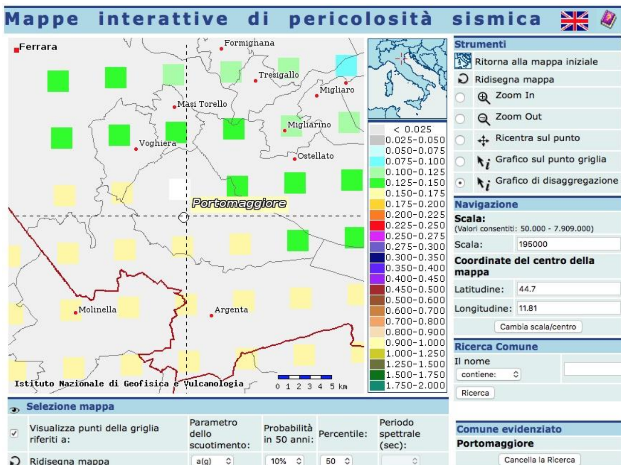
Fig. 5/12: Ubicazione dell'area in esame per lo studio di disaggregazione, per CU II .
