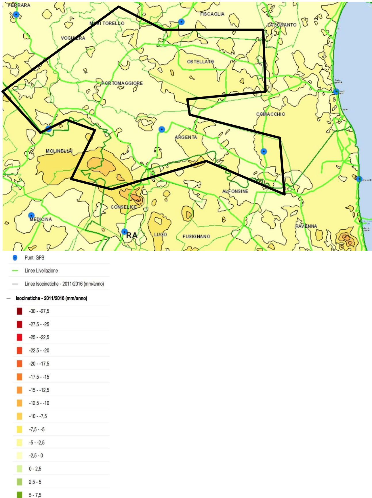
Fig. 4/2: Carta delle curve di eguale velocità di abbassamento del suolo (cm/anno) campagna di misura ARPAE periodo 2011- 2016
