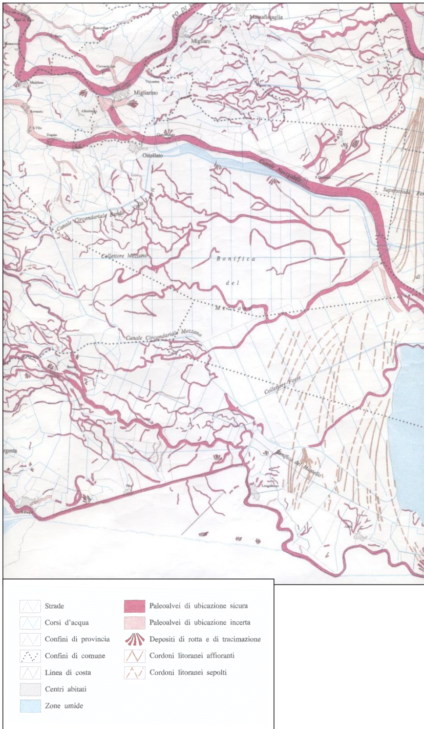
Fig. 2/10: Stralcio/dettaglio a Scala Libera della carta geomorfologica della provincia di Ferrara, porzione est.
