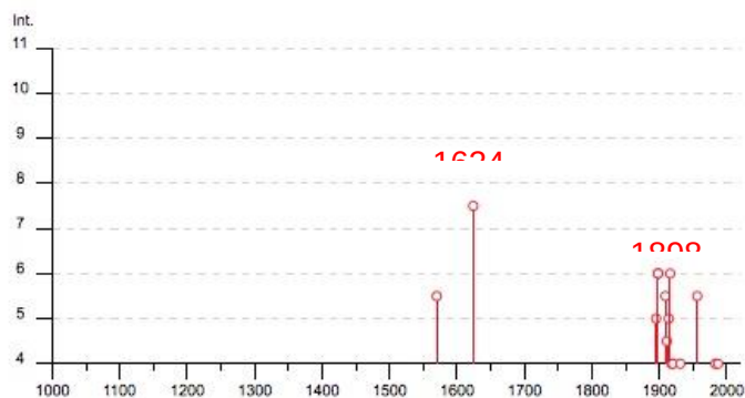
Fig. 5/11: storia sismica del Comune di Portomaggiore, L'Intensità Sismica (Is) massima registrata è pari a 7,5.
