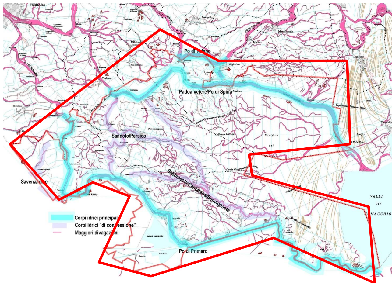
Fig. 2/2: Stralcio a Scala Libera della Carta Geomorfologica della Provincia di Ferrara (modificata dallo scrivente) nella quale sono rappresentati i corsi idrici principali e “secondari” come descritti in precedenza.
