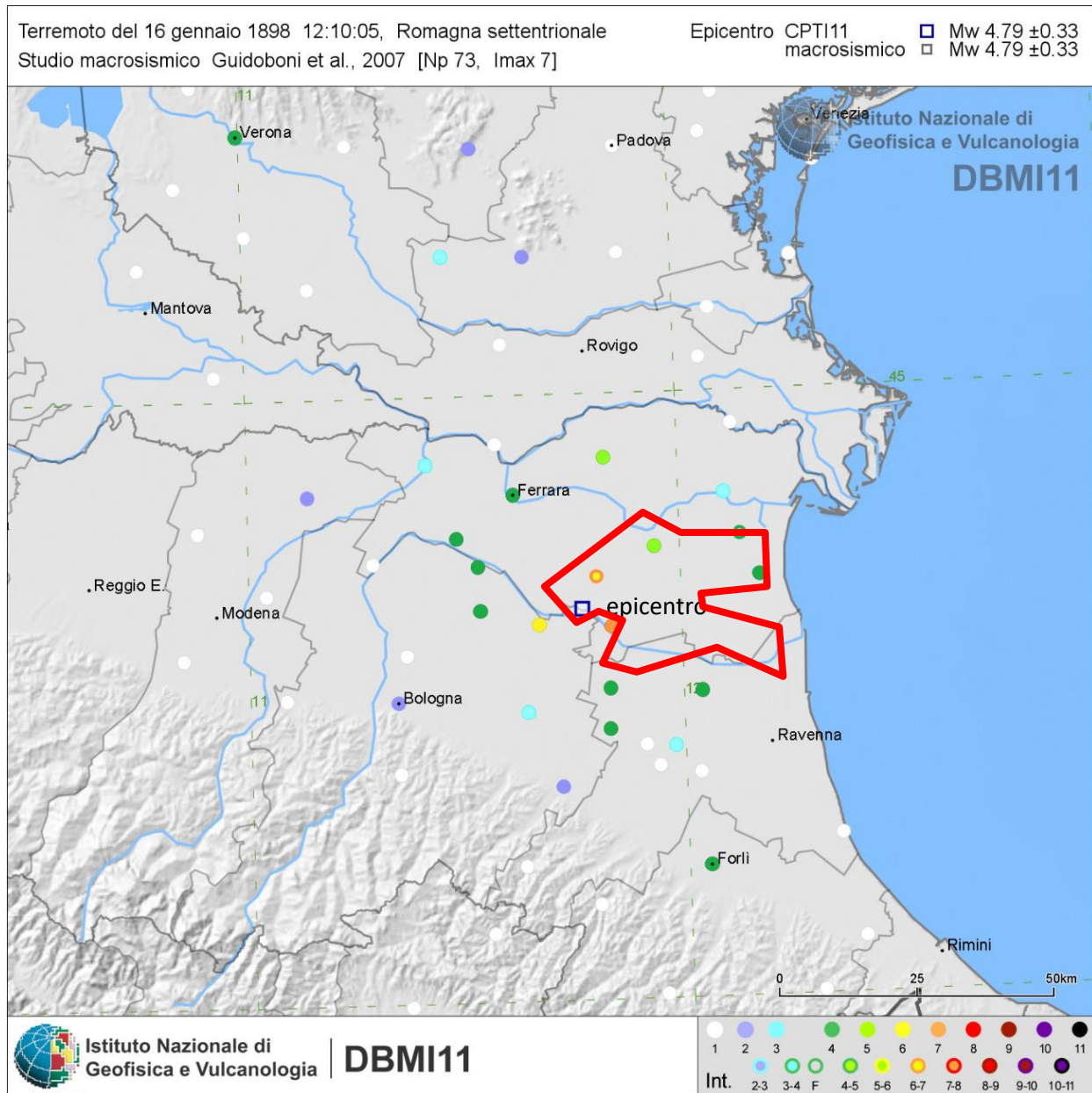
Fig. 5/9: evento del 1898: Romagna Settentrionale. Scala Libera, epicentro ed area in esame.
