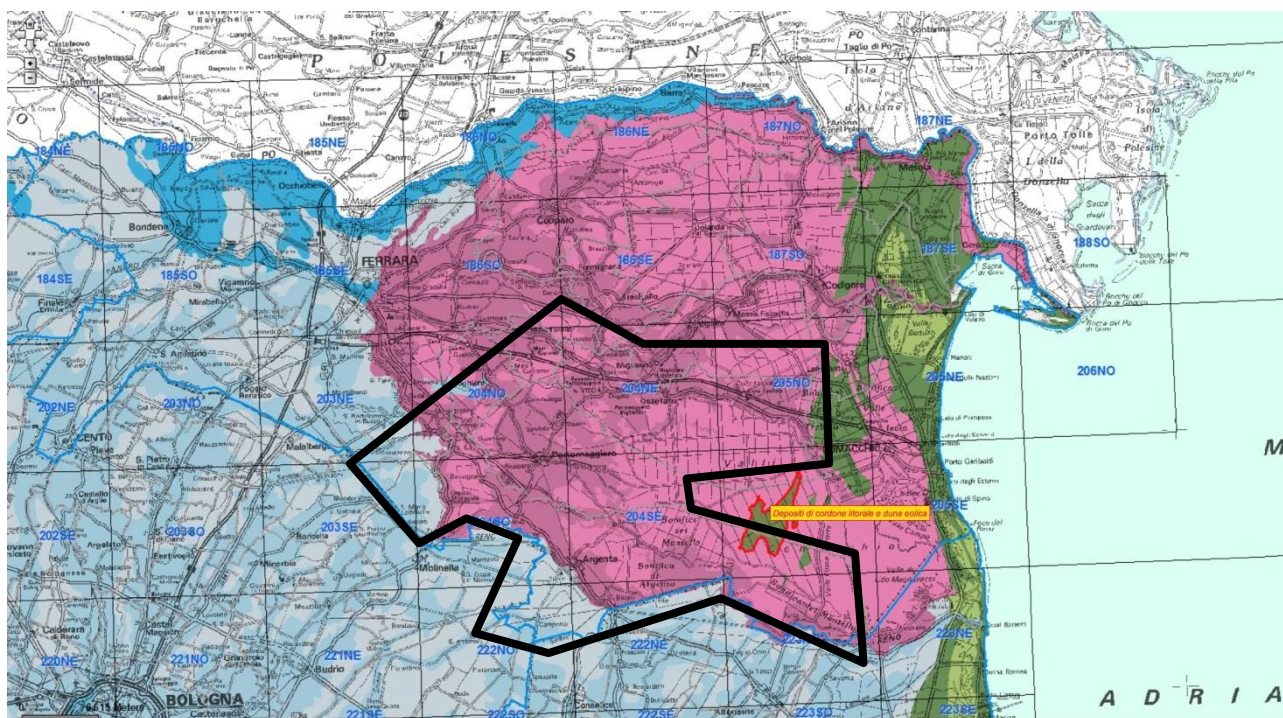
Fig. 3/4: Stralcio di Cartografia Geologica regionale (base al 250 000). Scala Libera. Sono evidenziati in rosso i Depositi di cordone litorale e dune eoliche.
