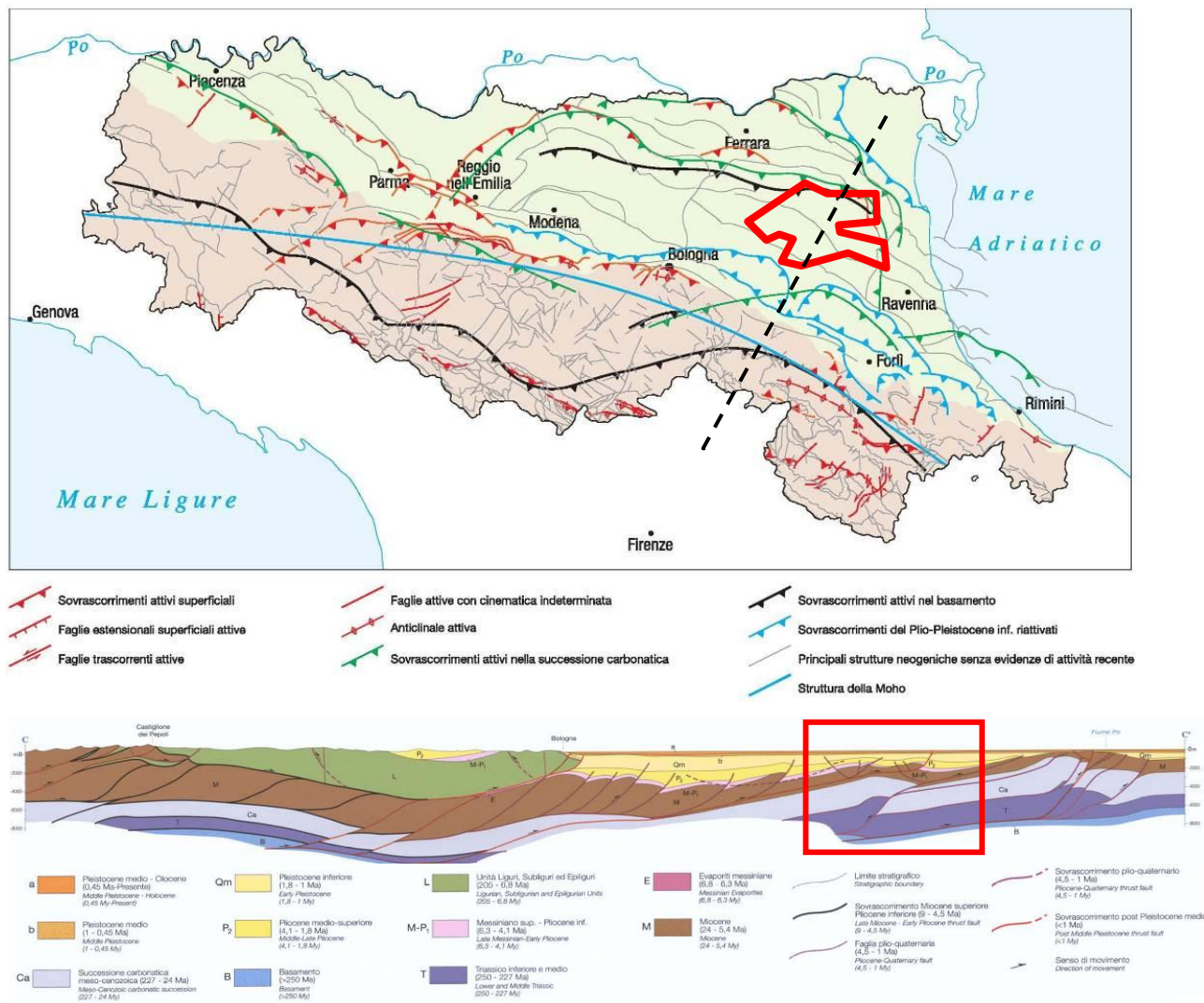
Fig. 1/1: Schema geologico profondo esemplificativo della Pianura Padana e relativa Sezione geologica esplicativa. Sono riportati gli andamenti delle pieghe e delle faglie del substrato e la traccia della medesima sezione.
