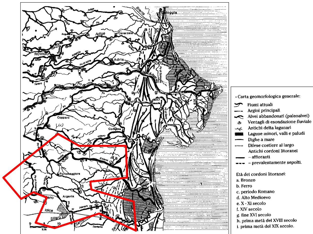
Fig. 2/1: Stralcio a Scala Libera dell'evoluzione geomorfologica della Pianura Ferrarese ad opera di M. Bondesan (1999), sono rappresentati i corsi principali del Grande delta del Po ed i territori dell'Unione, sono rappresentati altri elementi idraulici e le età delle posizioni della costa.
