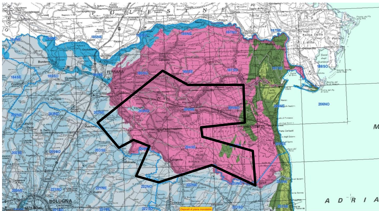
Fig. 3/1: Stralcio di Cartografia Geologica regionale (base al 250 000). Scala Libera. Le deposizioni individuate nelle tonalità del viola indicano derivazione alpina delle deposizioni locali, ascrivibili al grande edificio del paleo Delta del Po; nelle tonalità azzurre sono riportate le deposizioni di derivazione appenninica infine nelle tonalità del verde sono riportate le dune eoliche.
