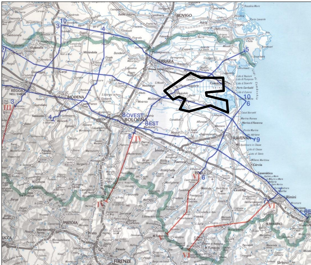
Fig. 6/15: Ubicazione dei profili idrostratigrafici relativi alle sezioni di cui di seguito. Scala Libera.
