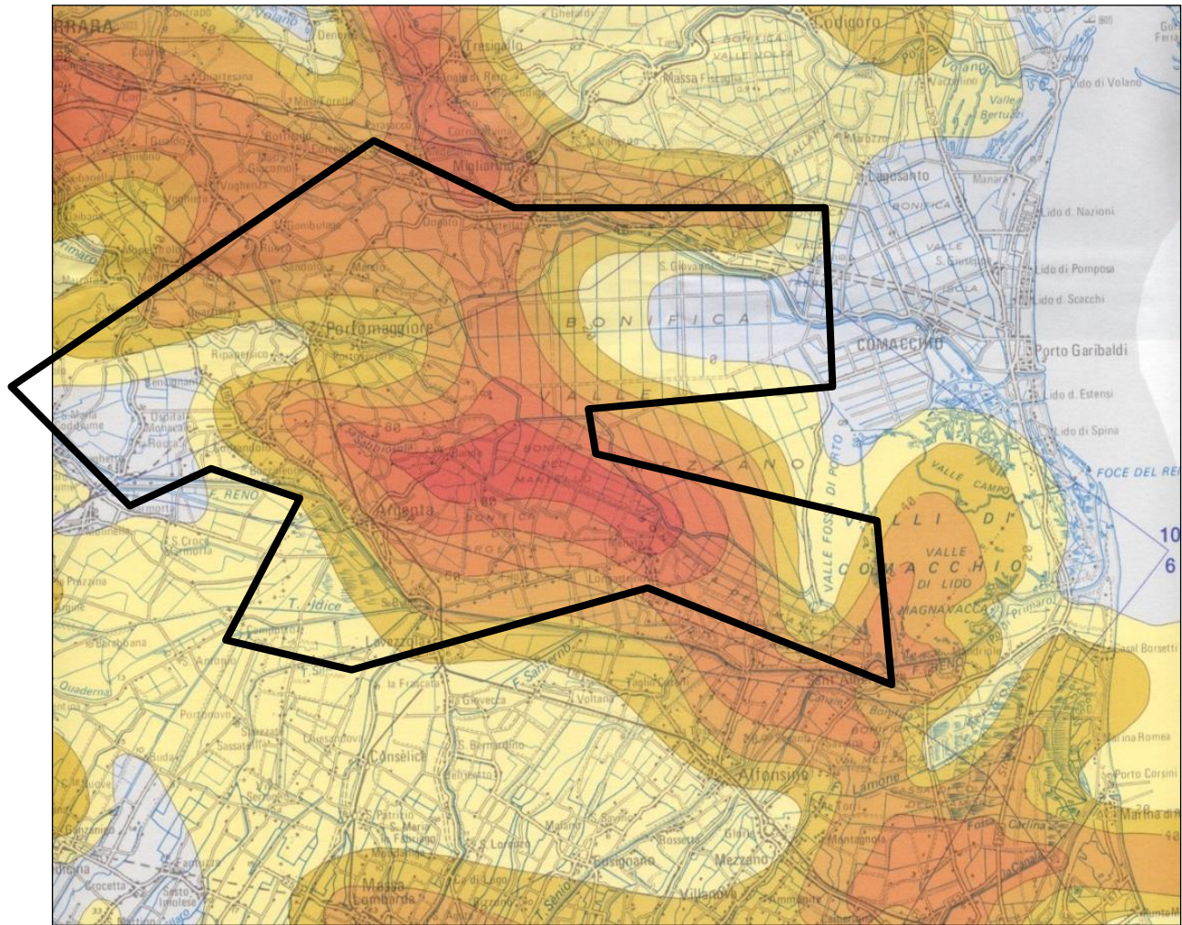
Fig. 6/20: Spessore cumulativo dell'acquifero A. Scala Libera.
