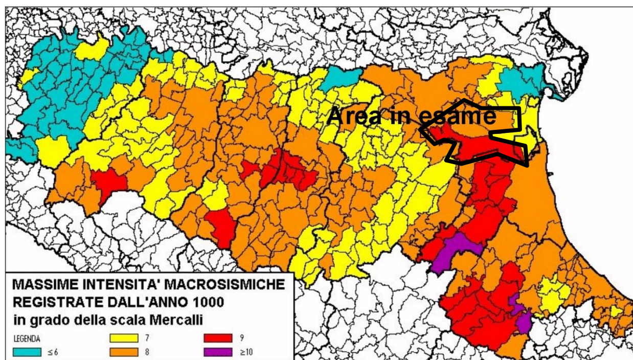
Fig. 5/20: Tavola a Scala Libera delle Massime Intensità Macrosismiche, dall'anno 1000.
