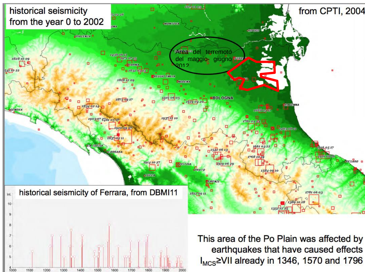
Figg. 5/5: Mappa degli epicentri dei terremoti avvenuti in Emilia- Romagna dal XIII sec. ad oggi per classi di magnitudo (CPTI 99). Scala Libera, la figura riporta come importante raffronto l'area del "cratere sismico" (come volgarmente ed imprecisamente denominato) dell'evento del maggio-giugno 2012.
