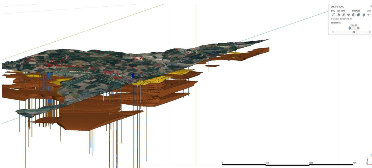
Fig. 1/6: Stralcio a Scala Libera rappresentativo delle possibilità di individuazione tridimensionale profonda Sezione Sud/Ovest-Nord/Est. Tratta dall'apposito sito web della Regione Emilia- Romagna. Il cono blu rappresenta l'abitato di Argenta.
