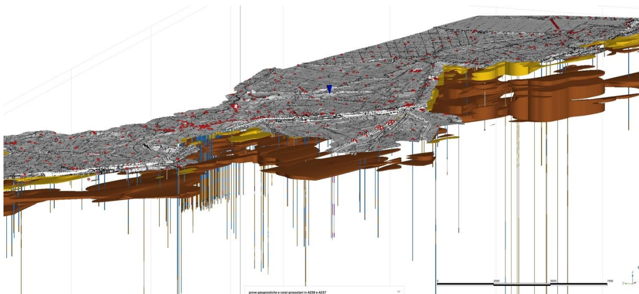
Fig. 1/4: Stralcio a Scala Libera rappresentativo delle possibilità di individuazione tridimensionale profonda dei "corpi grossolani" nei Gruppi AES8 e AES7. Tratta dall'apposito sito web della Regione Emilia- Romagna. Il cono blu rappresenta l'abitato di Argenta.
