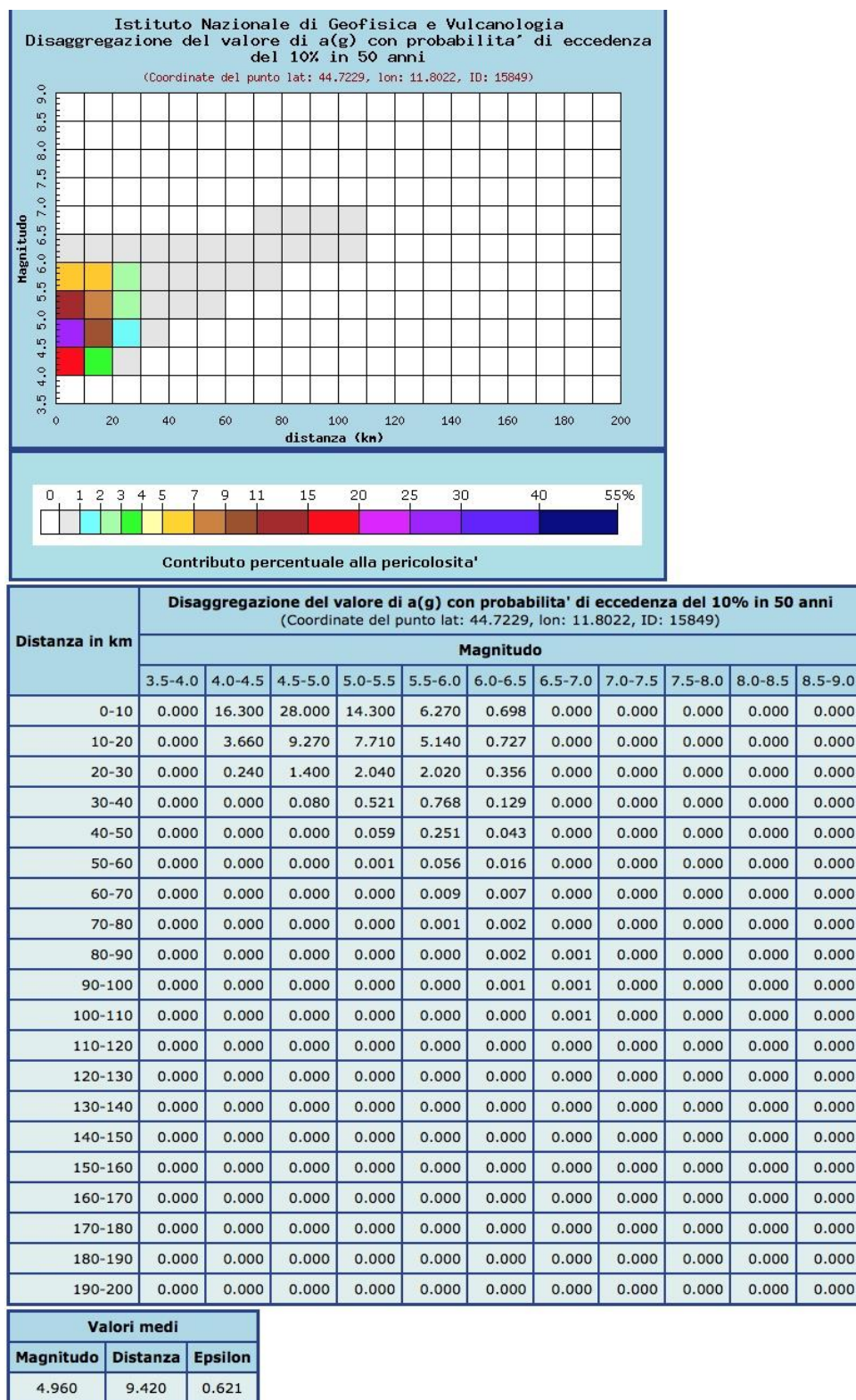
Figg. 5/13: tabelle di disaggregazione dei valori di M per l'area in esame (tratte dal sito del Progetto DPC-INGV- S1). La Magnitudo riportata   la Magnitudo Locale M_L (Richter) da non confondersi con la Magnitudo Momento M_W . Le due scale misurano "oggetti" sostanzialmente diversi e sono quindi scarsamente comparabili. Il corrispondente valore di M_W pu  essere comunque inteso maggiore di 5, sulla base di correlazioni "qualitative" proposte da vari Autori. Per il caso in esame il valore di M sarebbe pari a 5,21: M_W = 0,953M_L + 0,422 ; 3,9 \leq M_L \leq 6,8 (Yenier, Erdogan, Akkar- 2008), oppure pari a 5,22: M_W = 0,812M_L + 1,145 ; (INGV, 2004). Si osservi che tali valori sono validi solo per CU (Classe d'Uso) II .
