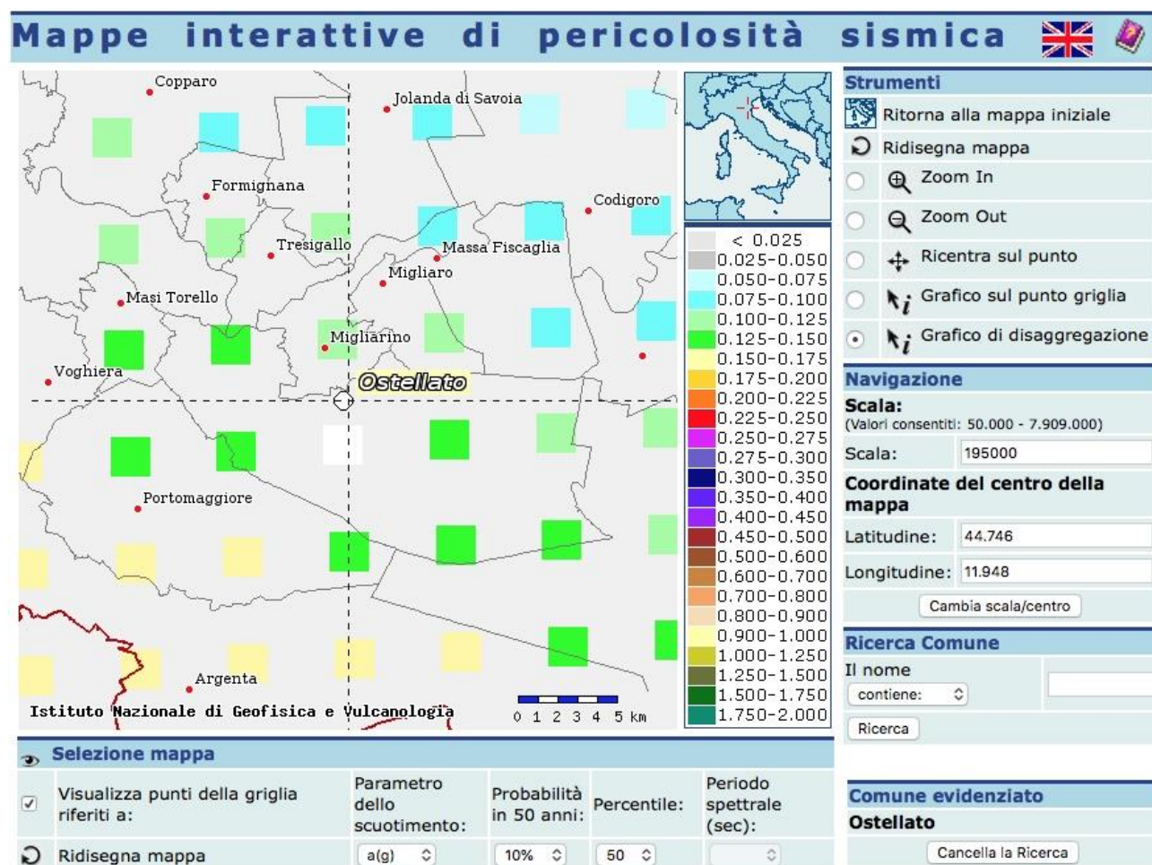
Fig. 5/10: Ubicazione dell'area in esame per lo studio di disaggregazione, per CU II.
