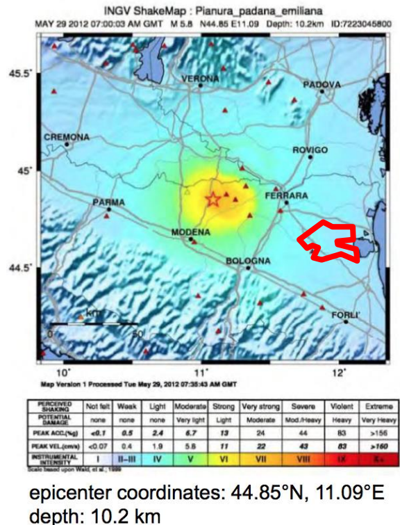
Fig. 5/19: Ubicazione degli epicentri degli eventi del 29 maggio 2012 e sviluppo areale delle relative intensità; il quadratino riporta l'area in esame, Scala libera (immagini tratte da L. Martelli- SGS Regione Emilia- Romagna; 7th Euregeo, Bologna 12- 15 Giugno 2012). Scala Libera.
