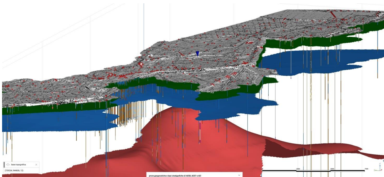
Fig. 1/3: Stralcio a Scala Libera rappresentativo delle possibilità di individuazione tridimensionale profonda dei Gruppi AES8, AES7 e AEI. Tratta dall'apposito sito web della Regione Emilia- Romagna. Il cono blu rappresenta l'abitato di Argenta.
