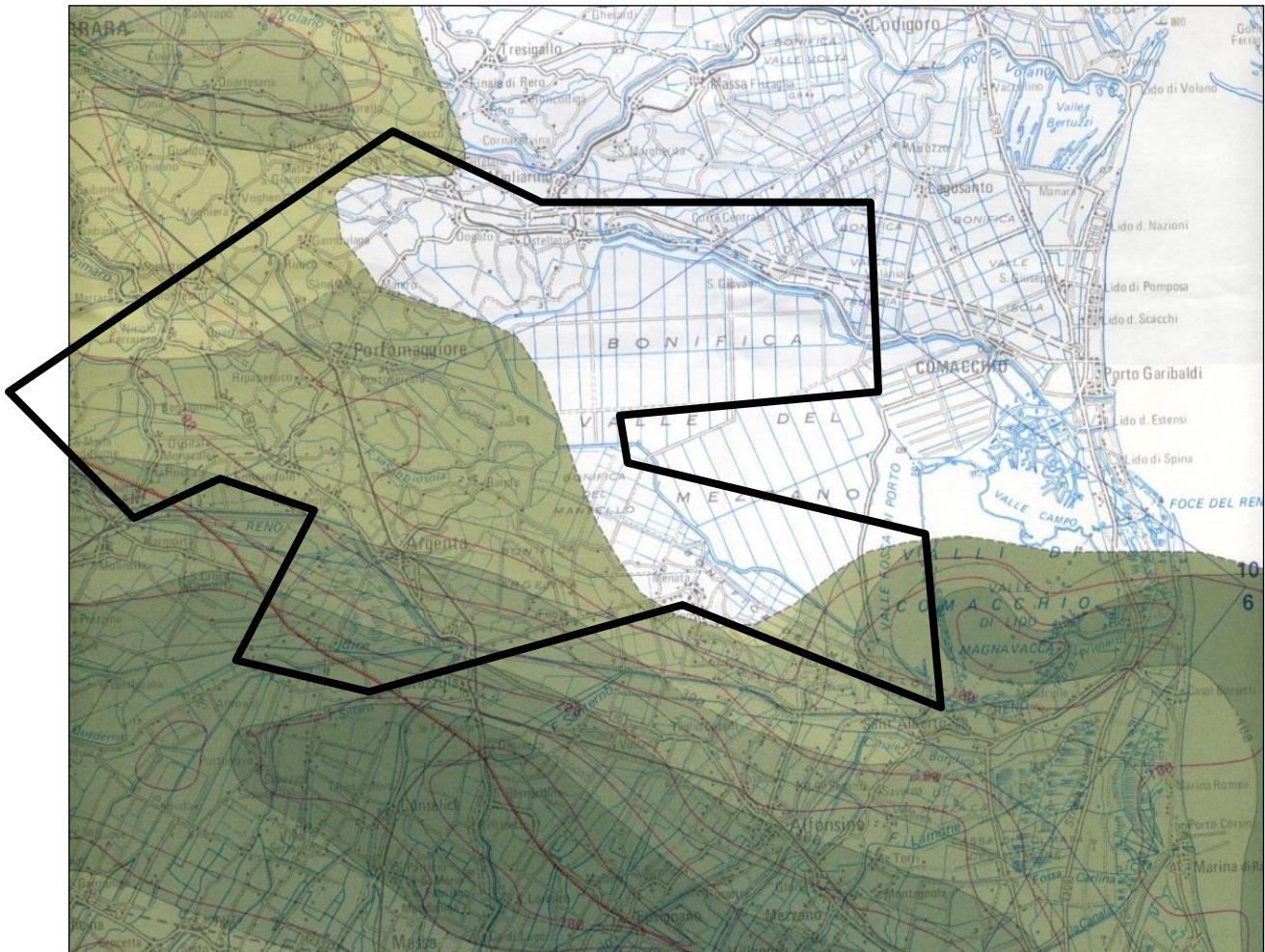
Fig. 6/19: Profondità del limite dell'acquifero B. Scala Libera.
