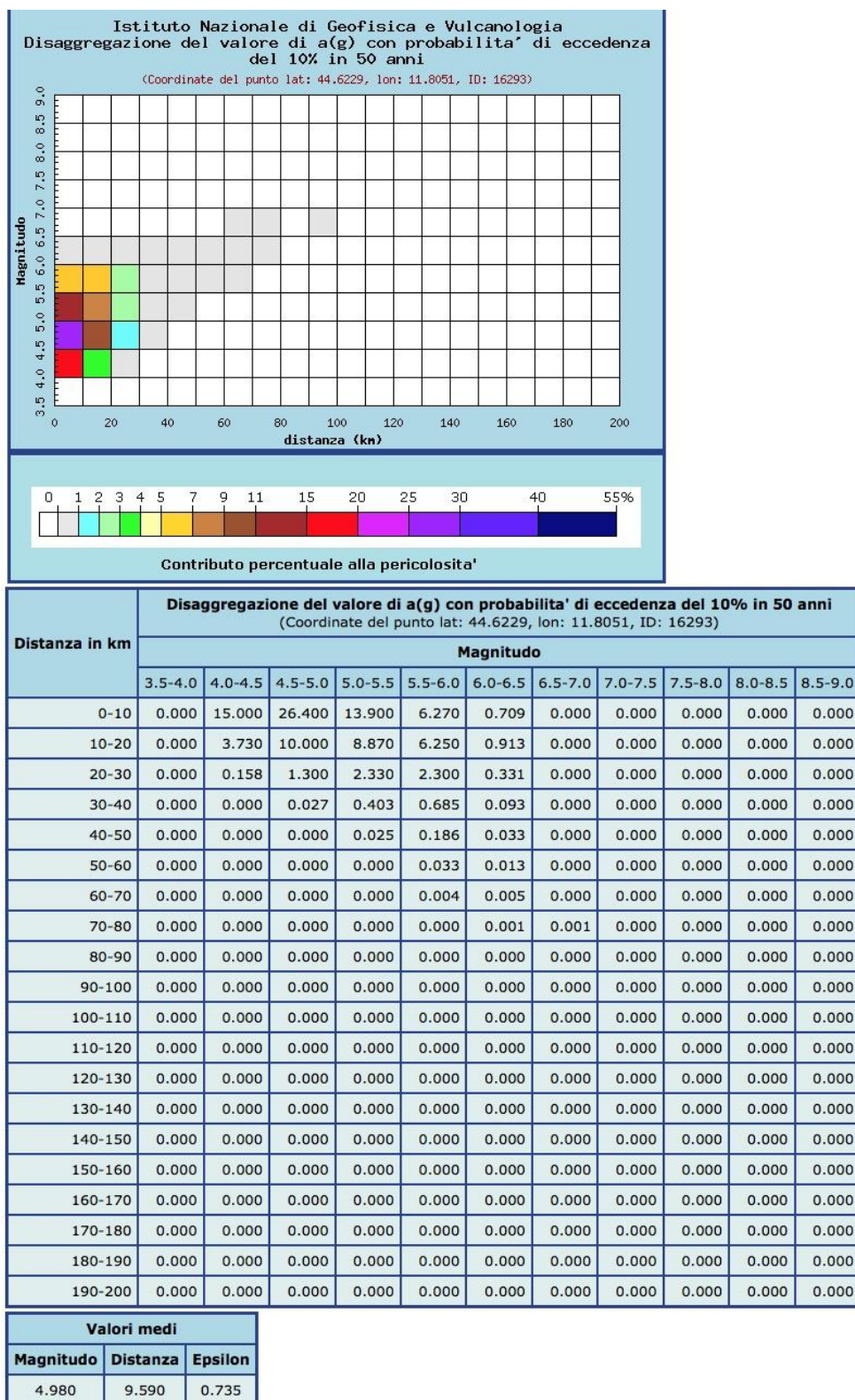
Fig. 5/9: tabelle di disaggregazione dei valori di M per l'area in esame (tratte dal sito del Progetto DPC-INGV- S1). La Magnitudo riportata   la Magnitudo Locale M_L (Richter) da non confondersi con la Magnitudo Momento M_W . Le due scale misurano "oggetti" sostanzialmente diversi e sono quindi scarsamente comparabili. Il corrispondente valore di M_W pu  essere comunque inteso maggiore di 5, sulla base di correlazioni "qualitative" proposte da vari Autori. Per il caso in esame il valore di M sarebbe pari a 5,21:
