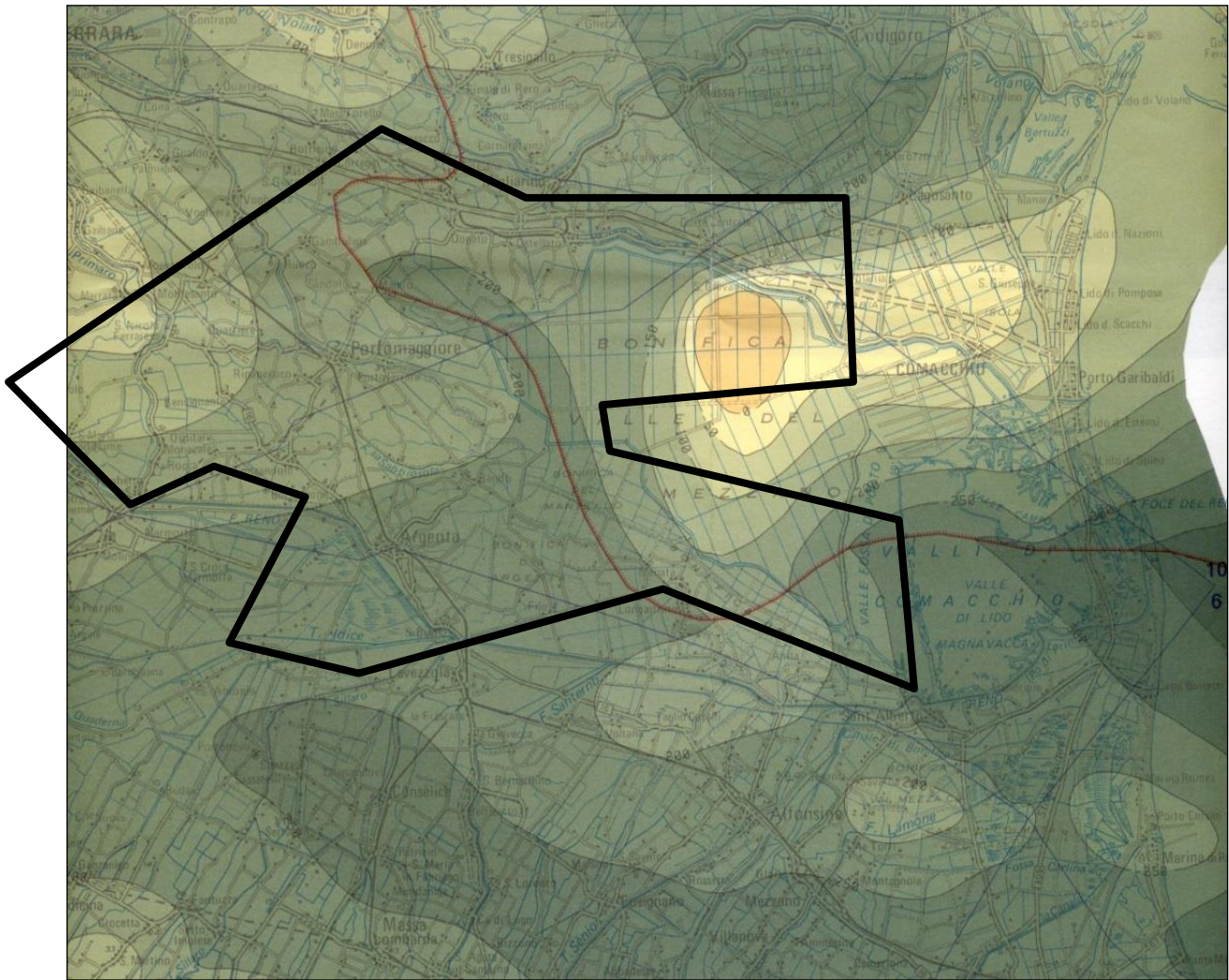
Fig. 6/18: Profondità del limite dell’acquifero A. Scala Libera.
