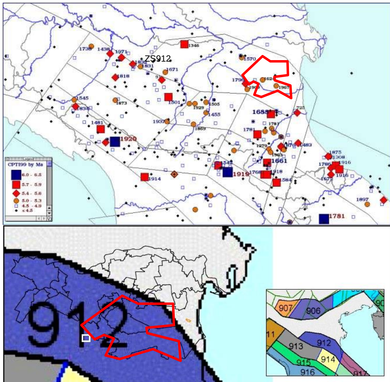
Figg. 5/4: Mappa degli epicentri dei terremoti avvenuti in Emilia- Romagna dal XIII sec. ad oggi per classi di magnitudo (CPTI 99). Scala Libera. Solo una modesta porzione (la porzione di Nord- Est) del Comune di Ostellato è esterna alla ZS 912. In merito alla individuazione delle ZS, queste sono relative all’assetto strutturale profondo. L’individuazione è ovviamente importante anche in relazione all’aspetto della Classificazione Sismica Nazionale di cui si dirà più oltre.
