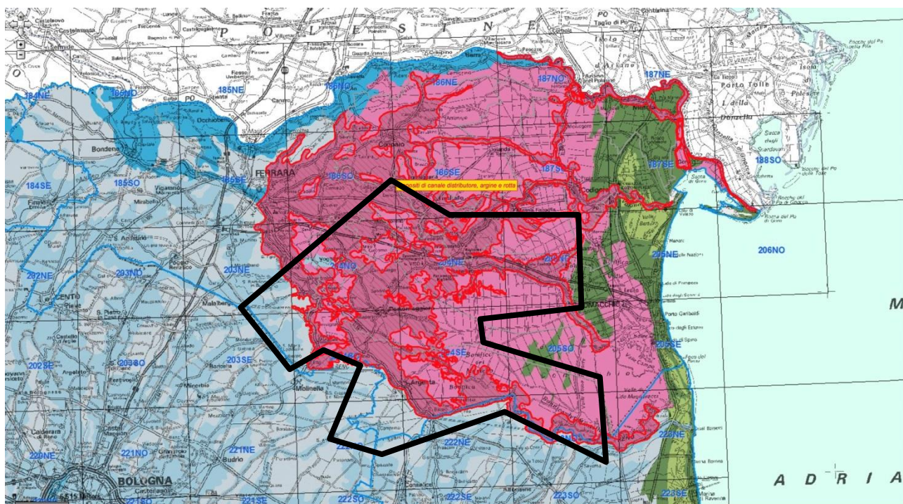
Fig. 3/2: Stralcio di Cartografia Geologica regionale (base al 250 000). Scala Libera. Sono evidenziati in rosso i Depositi di canale distributore, argine e rotta.
