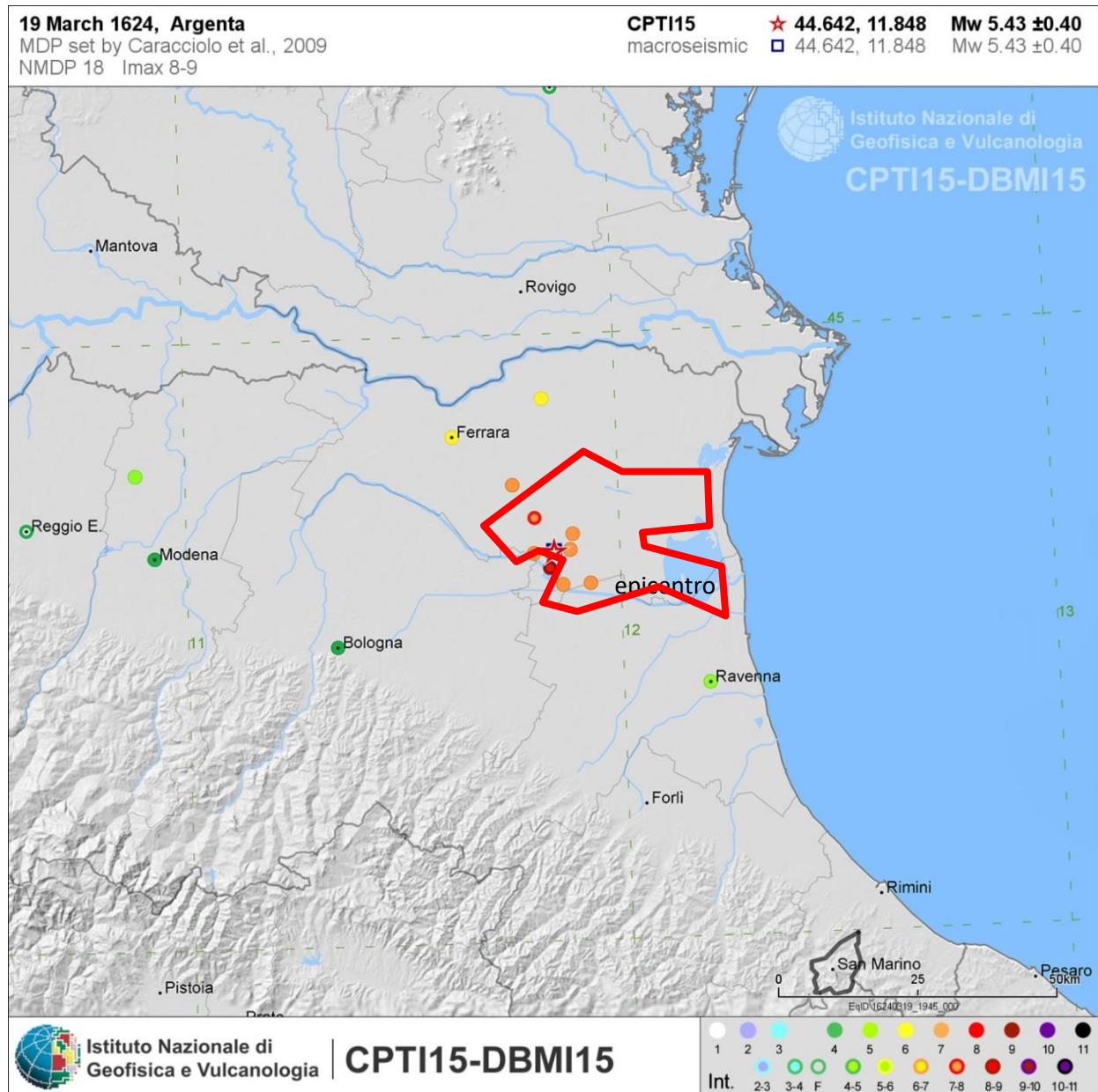
Fig. 5/12: evento del 1624: Argenta. Scala Libera, epicentro ed area in esame.
