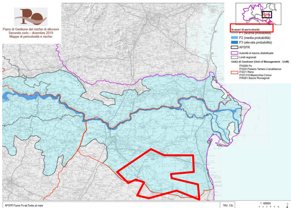
Tav. 6/5: Carta delle Aree Allagabili del Reticolo Principale Piano di Gestione del Rischio Alluvioni, Secondo Ciclo, Dicembre 2019. Scala Libera. Reticolo Principale, Fiume Po. P1
