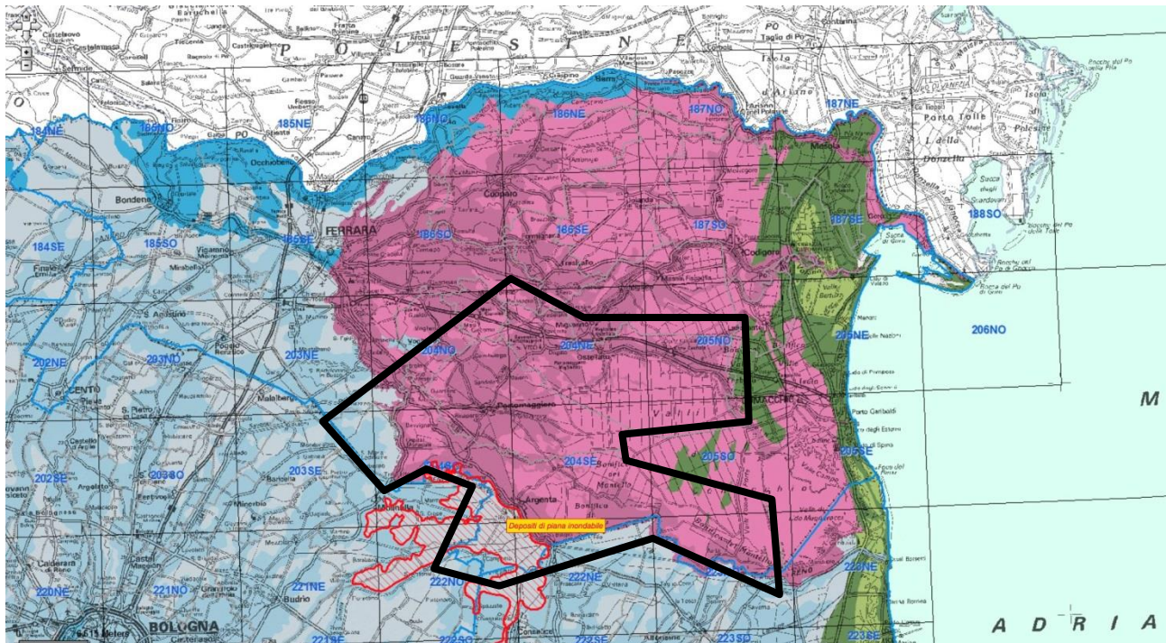
Fig. 3/6: Stralcio di Cartografia Geologica regionale (base al 250 000). Scala Libera. Sono evidenziati i Depositi di piana inondabile (nella fattispecie quelli presenti in destra Reno).
