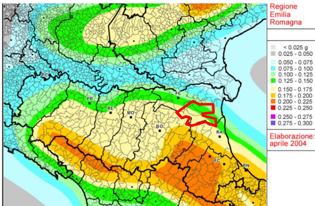
Fig. 5/22 Mappa di pericolosità sismica della Regione Emilia-Romagna espressa in termini di accelerazione massima al suolo con probabilità di eccedenza del 10% in 50 anni riferita a suoli rigidi (Cat. A). (Meletti & Montalbo, 2007).
