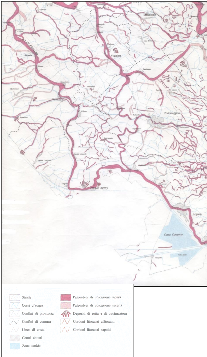
Fig. 2/11: Stralcio/dettaglio a Scala Libera della carta geomorfologica della provincia di Ferrara, porzione Ovest.
