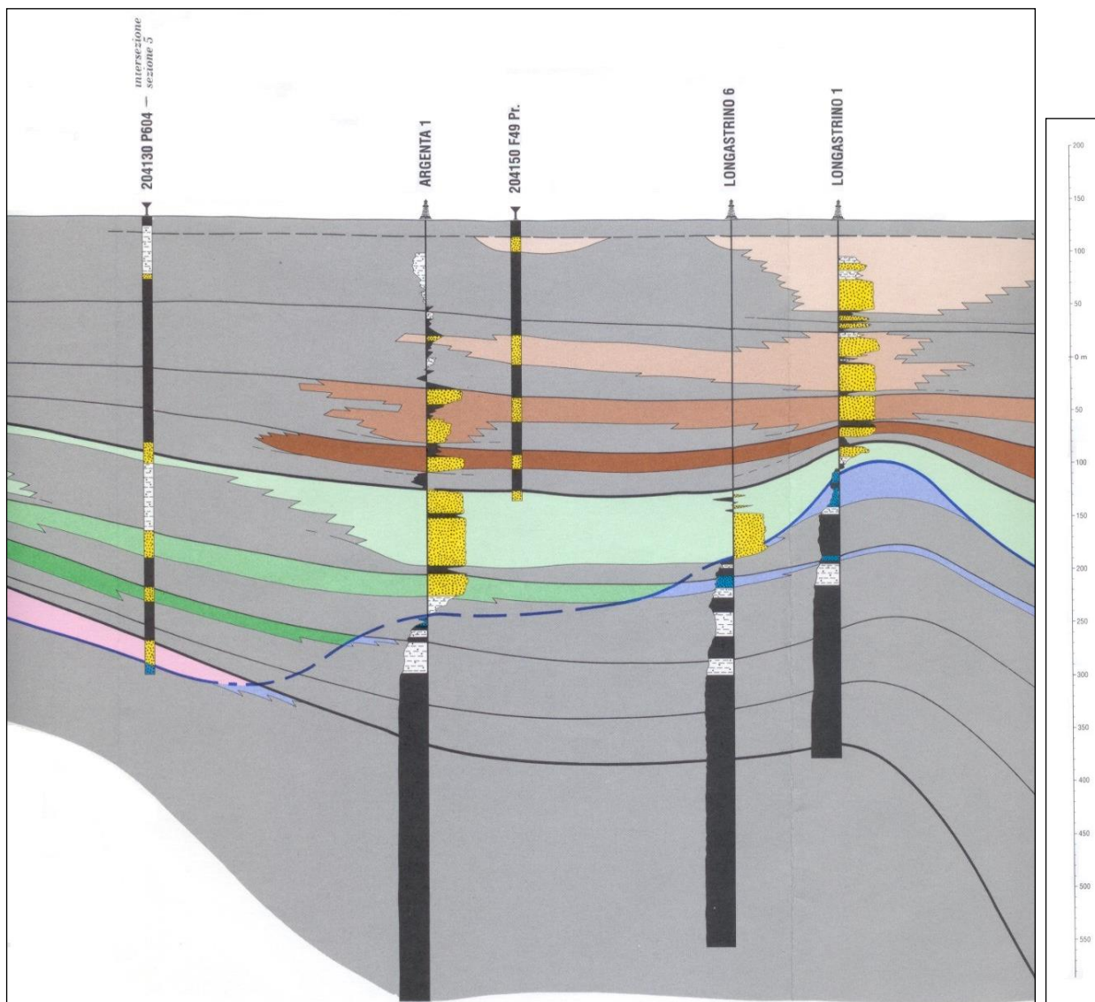
Fig. 6/17: Sezione idrostratigrafica 9 (WNW- ESE). Scala Libera.
