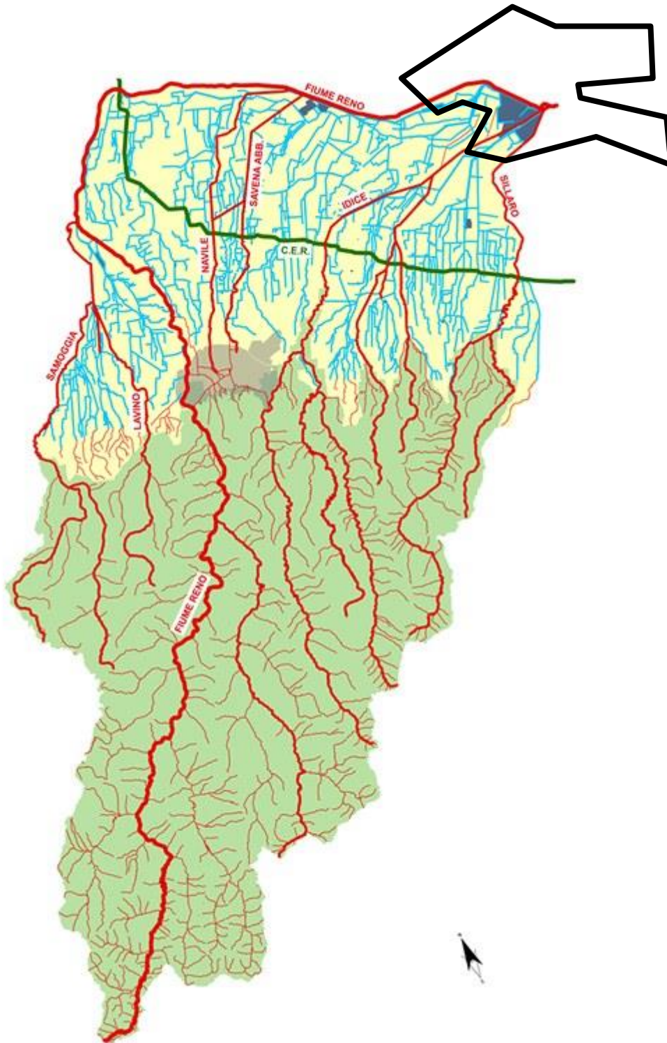
Fig. 6/3: rappresentazione a Scala Libera del bacino del Consorzio della Bonifica Renana. Si noti quanto sia estesa e come l'intero recapito avvenga in corrispondenza dell'Impianto Idrovoro del Saiarino/delle Valli di Argenta e Campotto.
