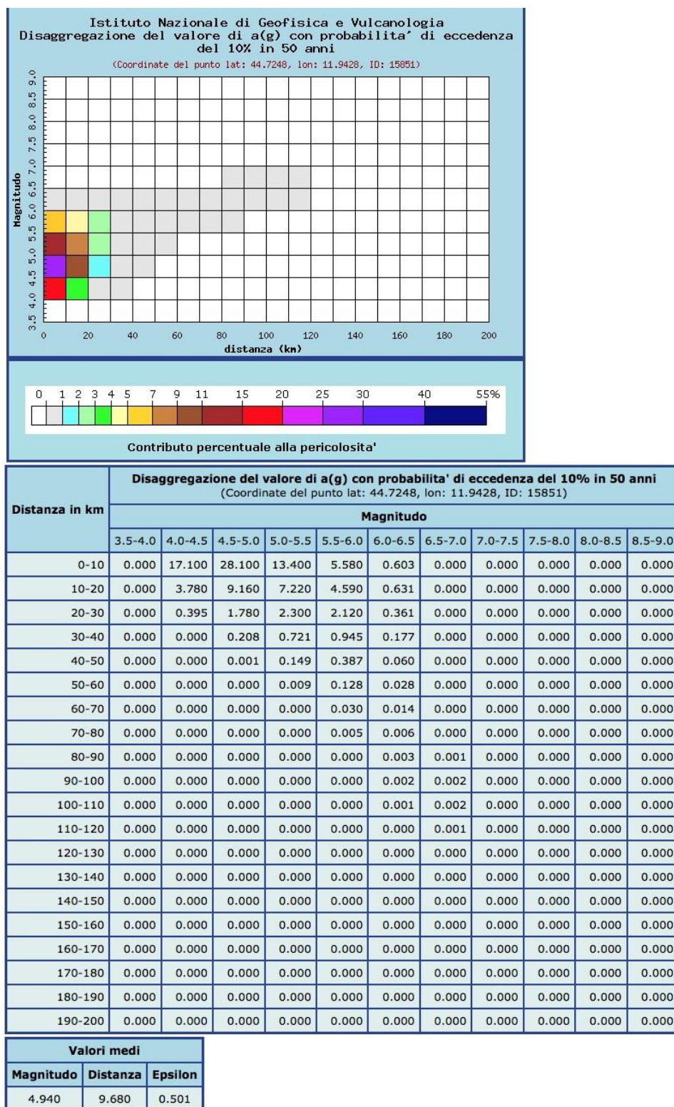
Figg. 5/11: tabelle di disaggregazione dei valori di M per l'area in esame (tratte dal sito del Progetto DPC-INGV- S1). La Magnitudo riportata   la Magnitudo Locale M_L (Richter) da non confondersi con la Magnitudo Momento M_w . Le due scale misurano "oggetti" sostanzialmente diversi e sono quindi scarsamente comparabili. Il corrispondente valore di M_w pu  essere comunque inteso maggiore di 5, sulla base di correlazioni "qualitative" proposte da vari Autori. Per il caso in esame il valore di M sarebbe pari a 5,21: M_w = 0,953M_L + 0,422 ; 3,9 \leq M_L \leq 6,8 (Yenier, Erdogan, Akkar- 2008), oppure pari a 5,22: M_w = 0,812M_L + 1,145 ; (INGV, 2004). Si osservi che tali valori sono validi solo per CU (Classe d'Uso) II .
