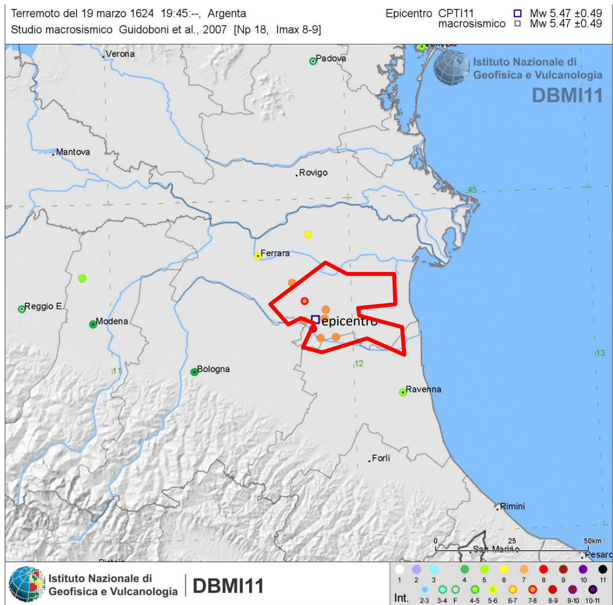
Fig. 5/8: evento del 1624: Argenta. Scala Libera, epicentro ed area in esame.
