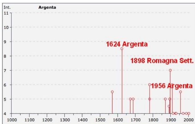
Figg. 5/7: storia sismica di Argenta, L'Intensità Sismica (Is) massima registrata è pari a 8,5.
