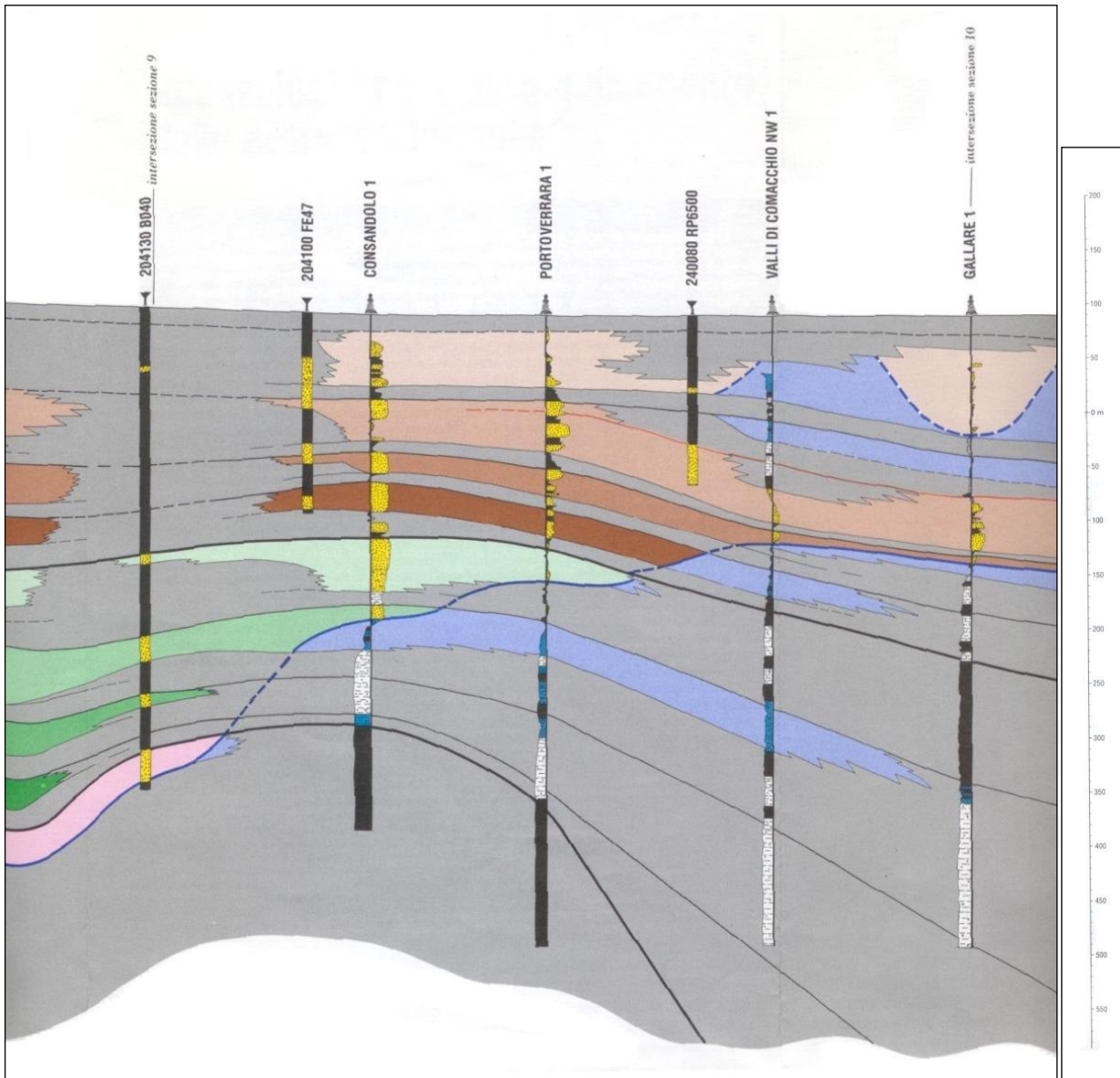
Fig. 6/16: Sezione idrostratigrafica 5 (SW- NE). Scala Libera.
