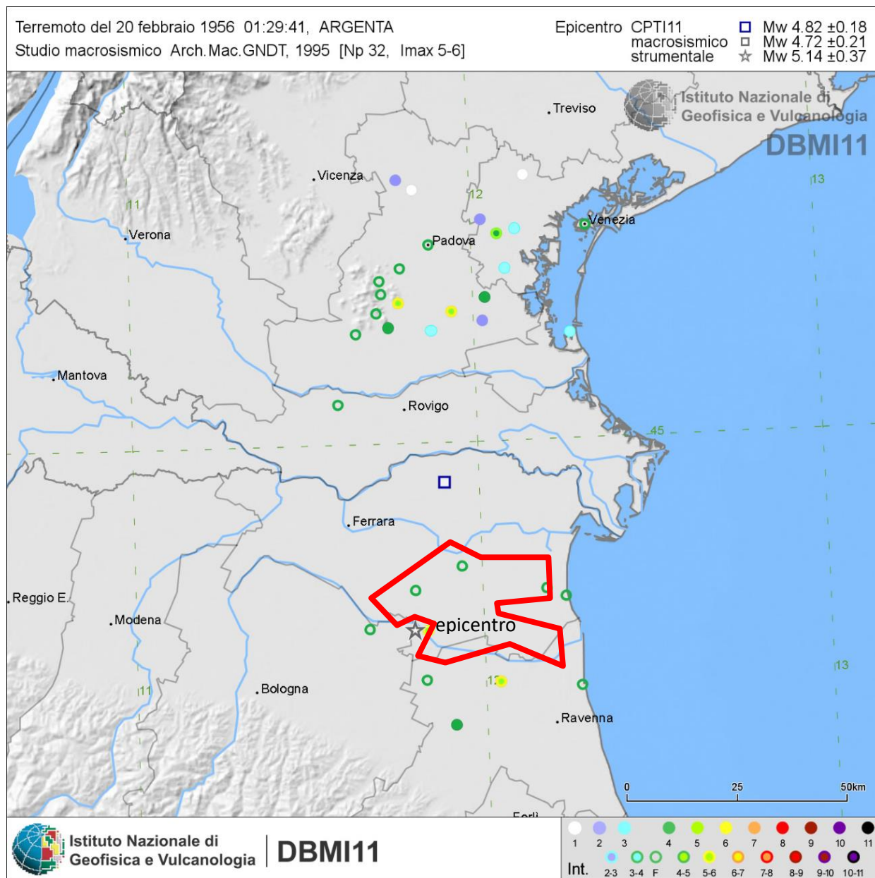
Fig. 5/10: evento del 1956: Argenta. Scala Libera, epicentro ed area in esame.
