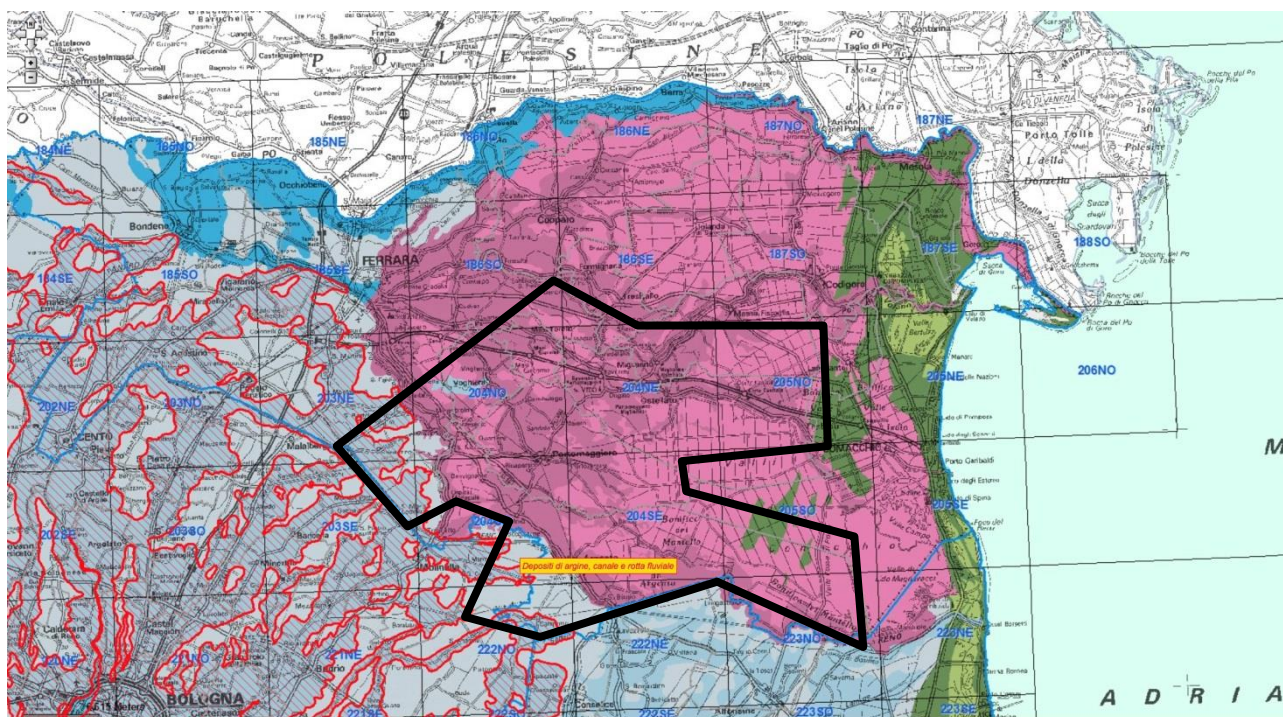
Fig. 3/5: Stralcio di Cartografia Geologica regionale (base al 250 000). Scala Libera. Sono evidenziati in rosso i Depositi di canale distributore, argine e rotta dei torrenti appenninici presenti in destra Reno.
