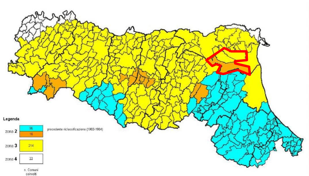
Fig. 5/21: Classificazione sismica del territorio regionale secondo l'OPCM 3274/2003. Il Comune di Argenta è evidenziato dal riquadro nero (colore arancione) è l'unico di ZS2 della Provincia di Ferrara.
