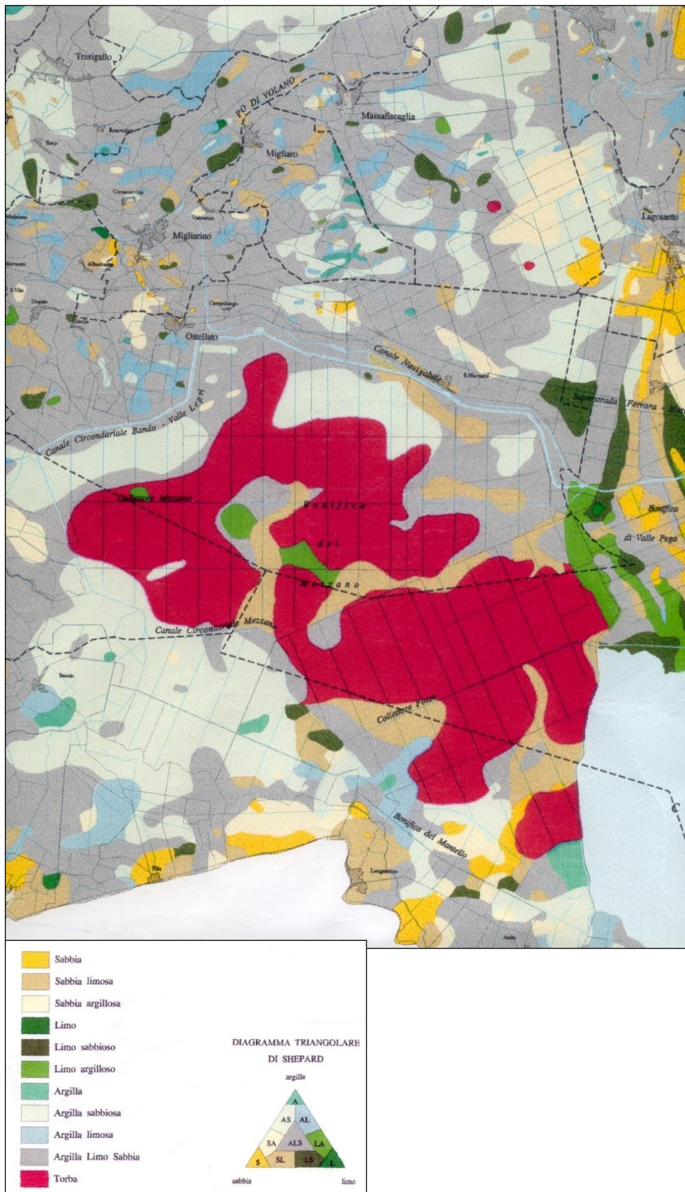
Fig. 3/19: Stralcio a Scala Libera della carta della litologia di superficie della Provincia di Ferrara, porzione Est.
