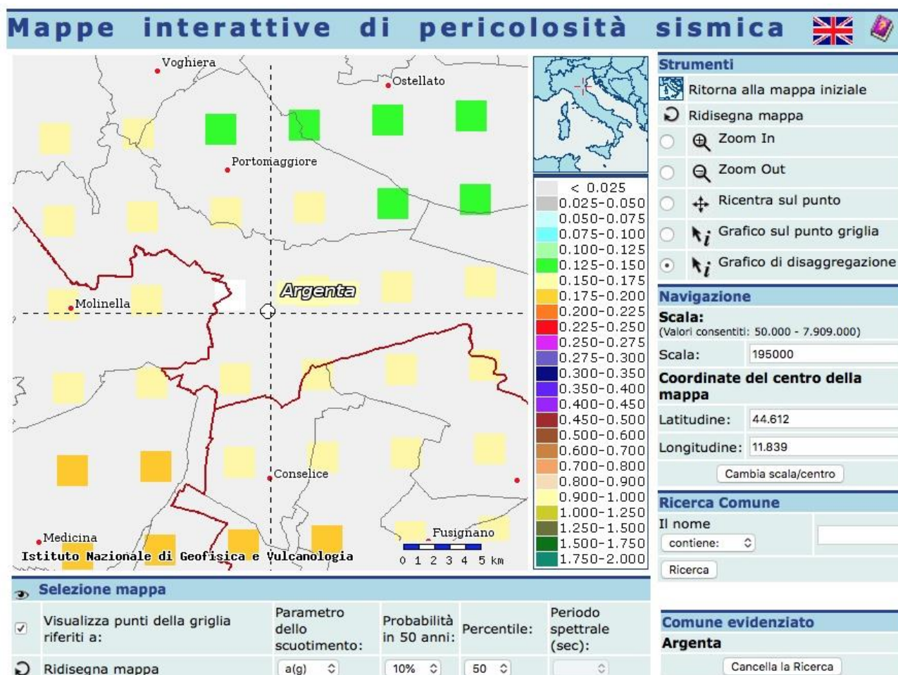
Fig. 5/8: Ubicazione dell'area in esame per lo studio di disaggregazione, per CU II .
