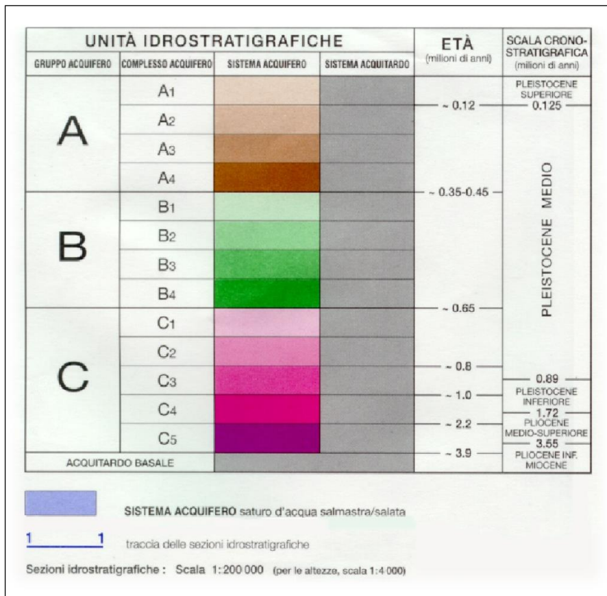
Fig. 6/15: Unità idrostratigrafiche della Pianura Padana Emiliano- Romagnola.
