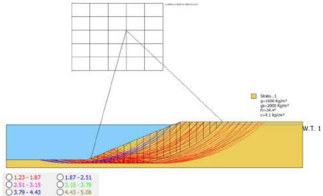
Superfici complessive calcolate raggruppate secondo intervalli di coefficiente di sicurezza.
