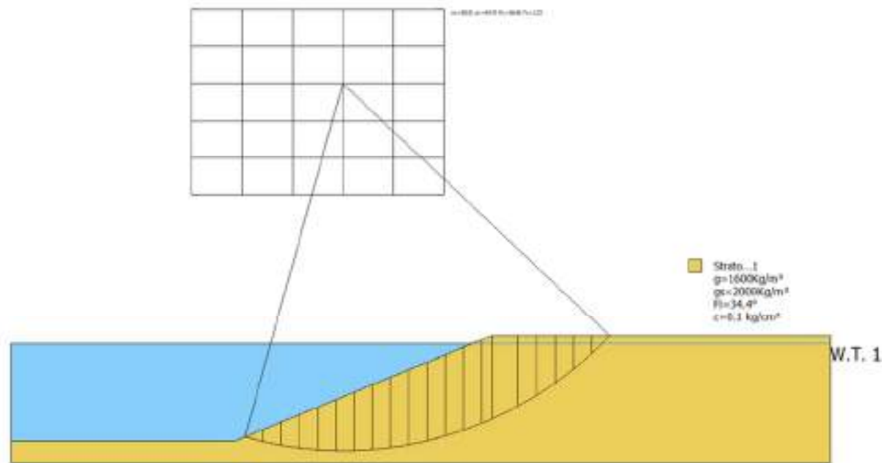
Definizione della superficie critica di progetto (a minor coefficiente di sicurezza).
