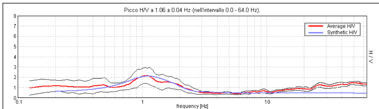
Figura 7 - confronto tra curva HVSR1 sperimentale registrata nel sito (scelta per il fit congiunto con prova MASW-Re.Mi.) e curva teorica (blu) relativa al modello di sottosuolo proposto per il sito.
