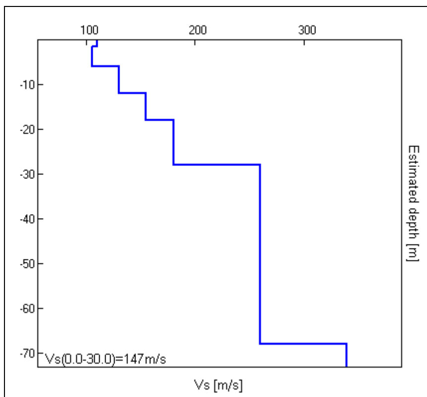
Figura 8 - Modello di velocità delle onde di taglio S (modello medio sotto il profilo effettuato) derivato da fit congiunto tecnica MASW-Re.Mi. e tecnica HVSr
