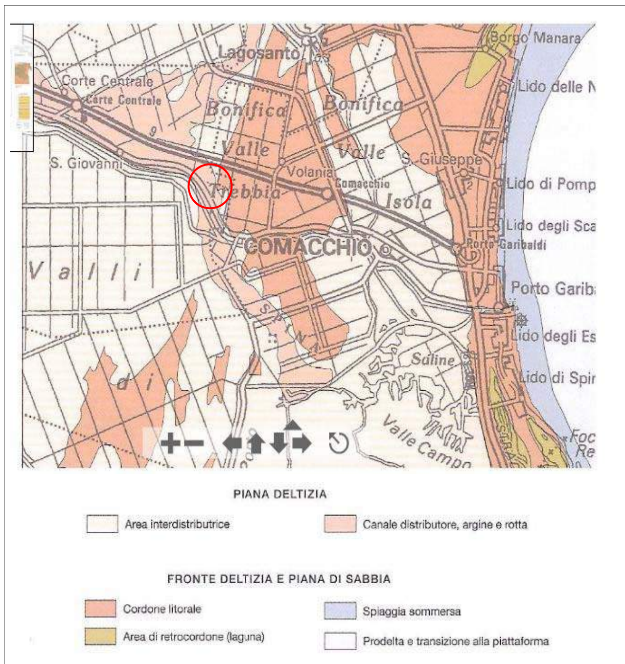
Schema degli ambienti deposizionali.
